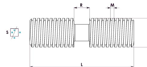
Verstellspindel Adjusting Screw Vis de réglage
